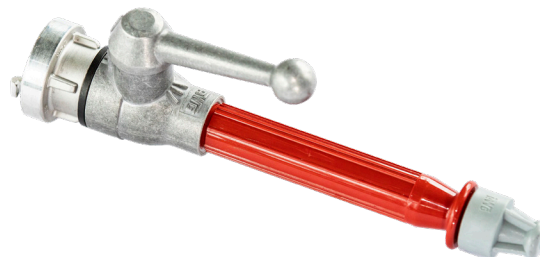
Abbildung 43: D-Mehrzweckstrahlrohr - 25 / 50 l/min Wurfweiten bis ca. 15 Meter.
