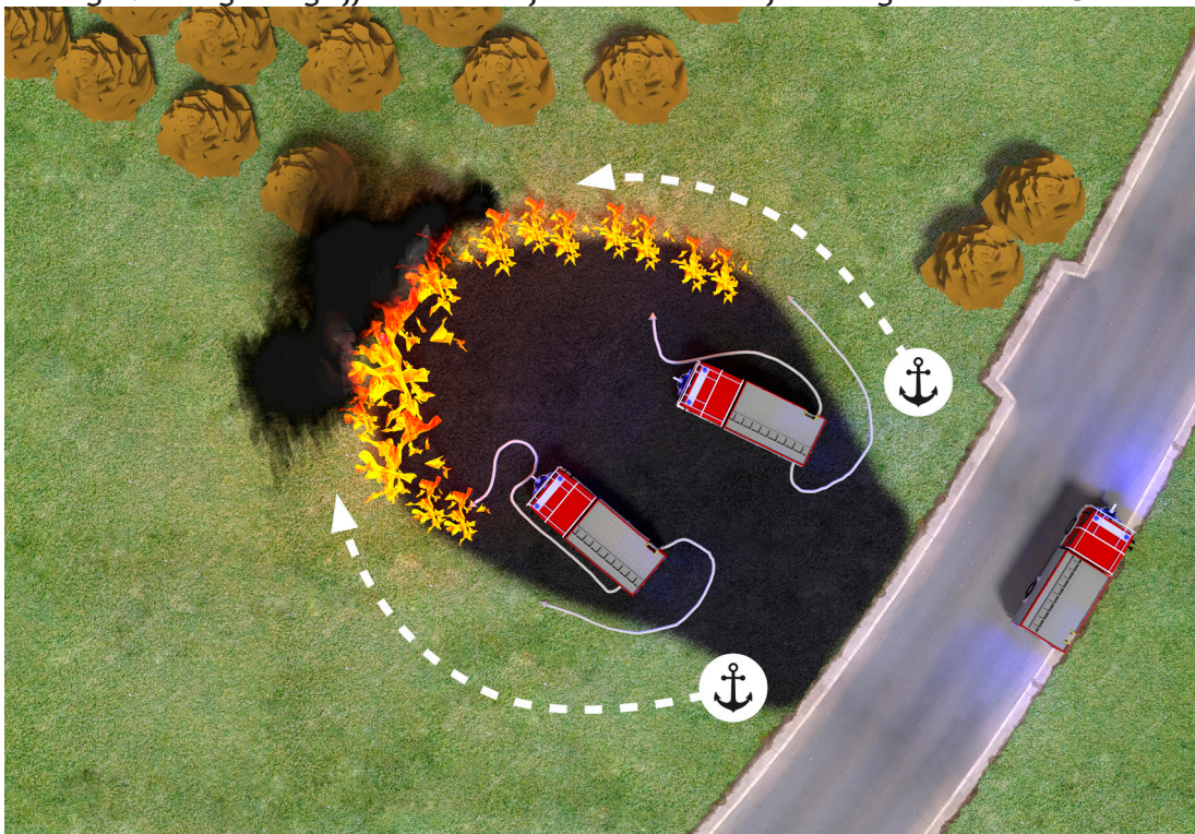
Abbildung 60: Zangenangriff mit wasserführenden Löschfahrzeugen aus dem Schwarzbereich
