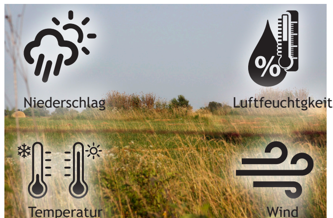
Abbildung 12: Relevante meteorologische Parameter
