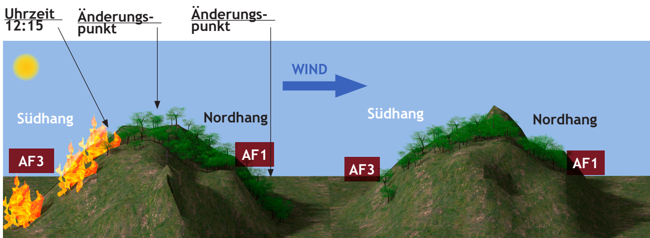
Abbildung 17: Einfache Waldbrandprognose
