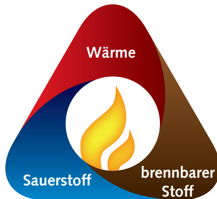
Abbildung 9: Verbrennungsdreieck
