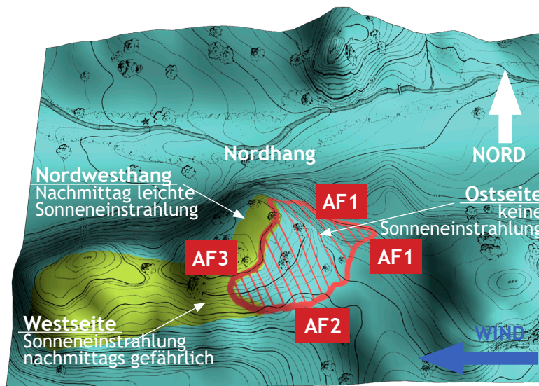
Abbildung 19: Einfache Waldbrandprognose
