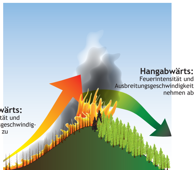
Abbildung 14: Hangneigung - Unterschiedliche Ausbreitungsgeschwindigkeit - Hangaufwärts bzw. Hangabwärts
