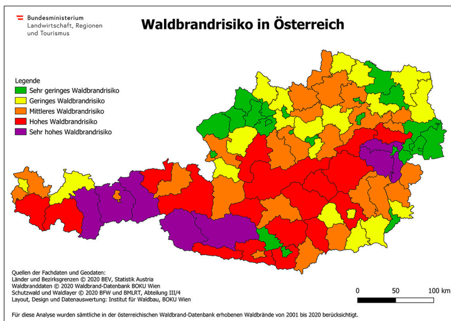
Abbildung 2: Österreichische Waldbrandrisikokarte (Stand 2020, Quelle: Universität für Bodenkultur Wien, https://fmlink.at/ites )
