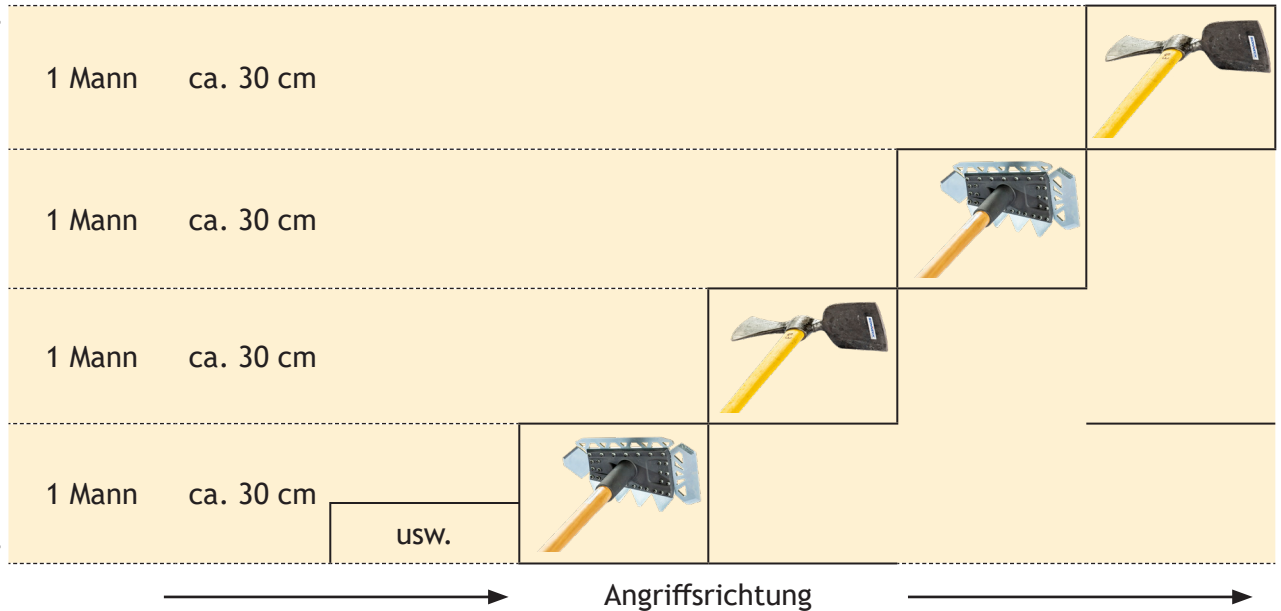
Abbildung 68: Geräte und personeller Aufwand einer defensiven Brandbekämpfung
