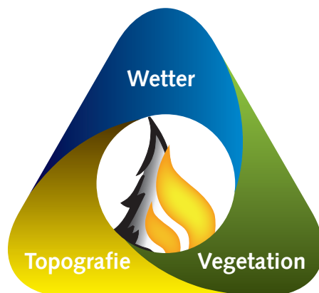
Abbildung 10: Vegetationsbrand-Verbrennungsdreieck
