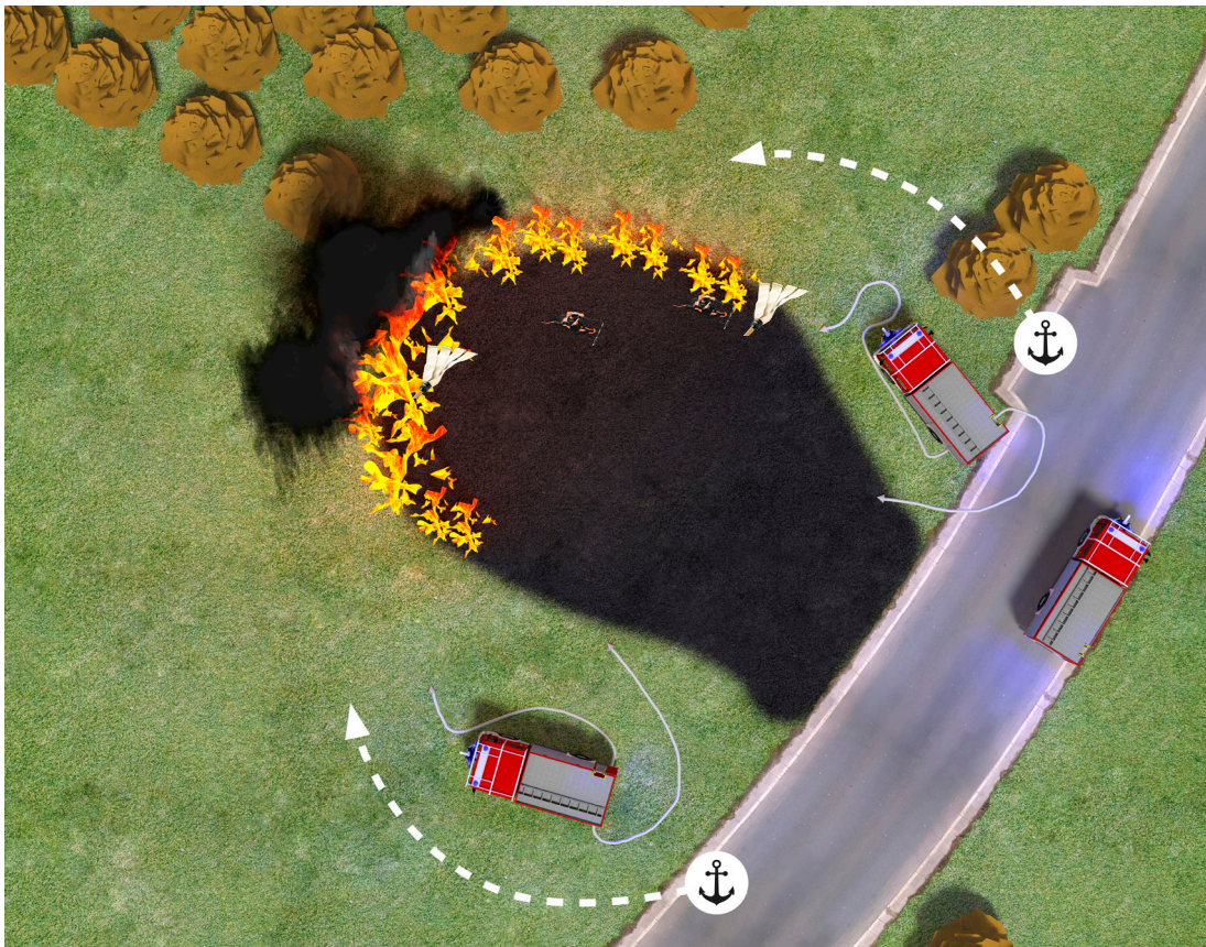
Abbildung 59: Zangenangriff mit wasserführenden Löschfahrzeugen aus dem Grünbereich
